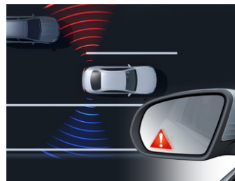
Totwinkel-Assistent (234) Dieser Assistent sieht für Sie genau hin: Das System kann Sie – insbesondere sobald Sie den Blinker betätigen – vor Seitenkollisionen mit anderen Verkehrsteilnehmern im toten Winkel warnen. Auch nach der Fahrt bleibt das System noch wachsam und warnt Sie, wenn Sie die Tür im falschen Moment öffnen. Ein wichtiger Schutz – vor allem für Fahrradfahrer.
